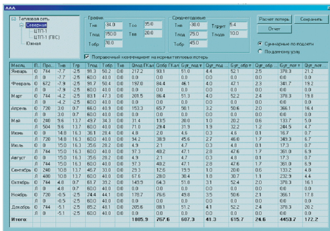
Рисунок 9.3 - Диалоговое окно расчета тепловых потерь
