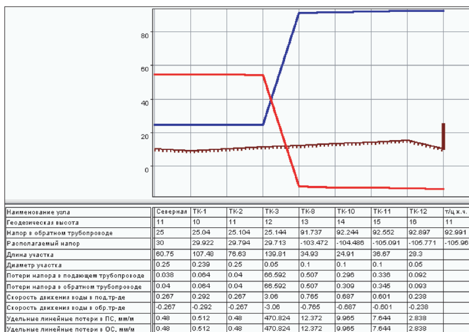
Рисунок 7.11 - Пьезометрический график
